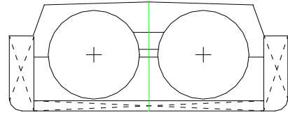
Type G, Ladingtanktoestand 1, (ook bij gladdek)
