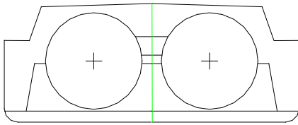
Type G, Ladingtanktoestand 1, Ladingtanktype 1 (ook bij gladdek)
