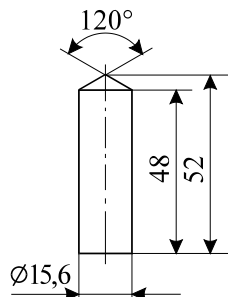
Fig 2: Cilindervormige bronzen zuiger; afmetingen in mm
