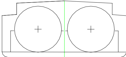
Type N, Ladingtanktoestand 2,3 of 4, Ladingtanktype 1 (ook bij gladdek)
