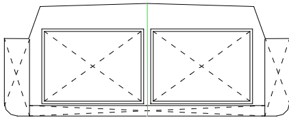
Type G, Ladingtanktoestand 2, Ladingtanktype 1 (ook bij gladdek)
