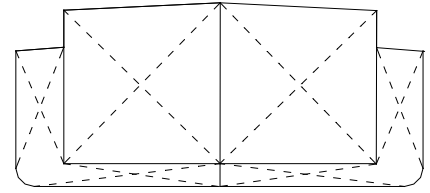
Type N, Ladingtanktoestand 2,3 of 4, Ladingtanktype 3 (ook bij gladdek)
